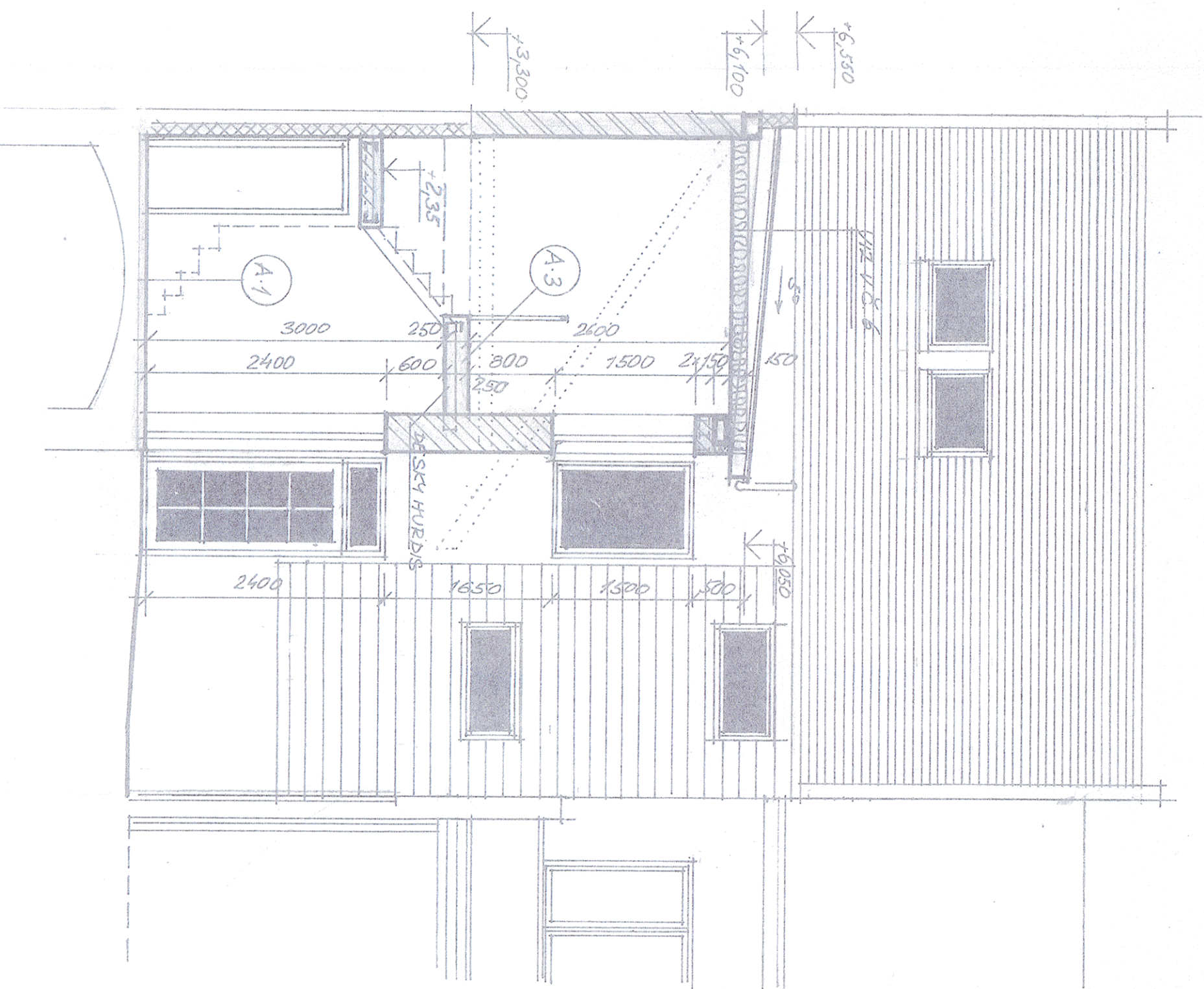
ŘEZ C-C', POHLED DVORNÍ 1:50
